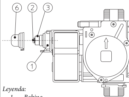
Válvula GAS SIT 845
